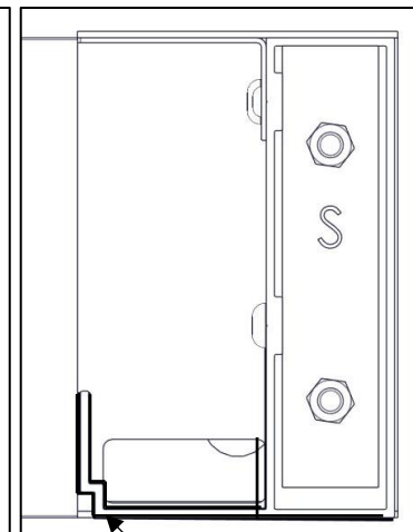
Etanchéité récupérateur
